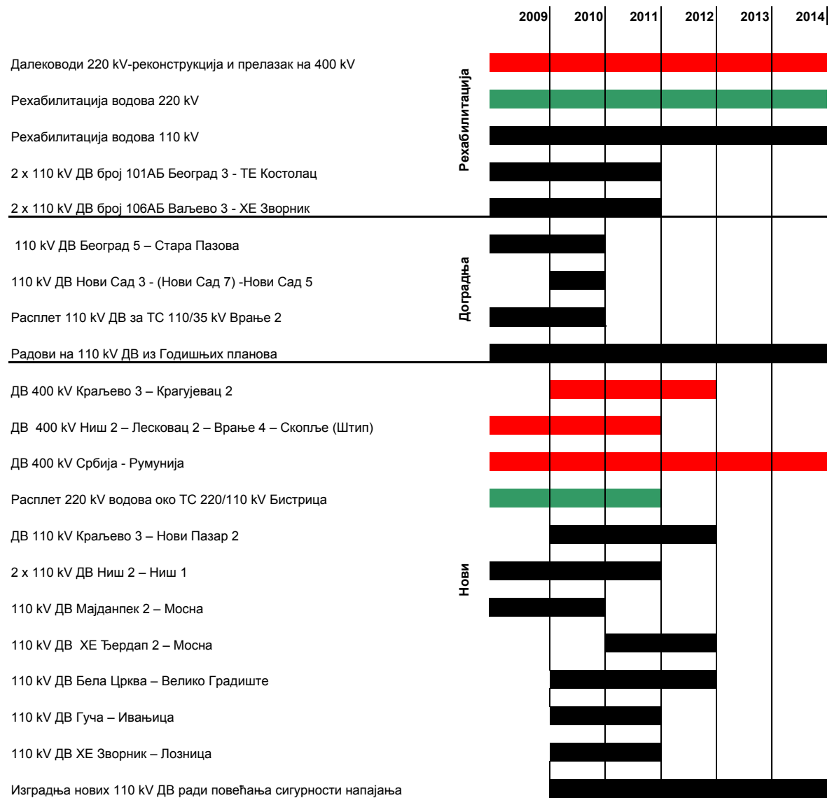
Сл.11.2. Рехабилитација, доградња и нови далеководи у периоду до 2014. године
